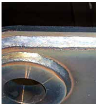
Exemplu de pozitionare corecta a sarmei
