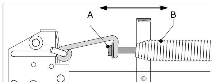
Fig. 6.5 Scharnier aan de muur-/kapzijde
