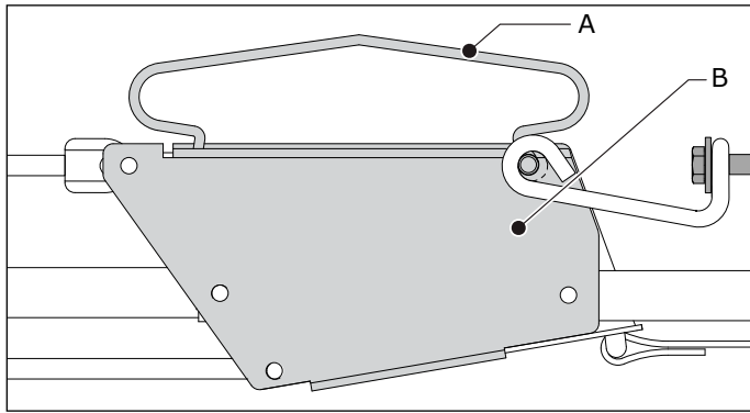
Abb. 4.7 Distanzfeder
