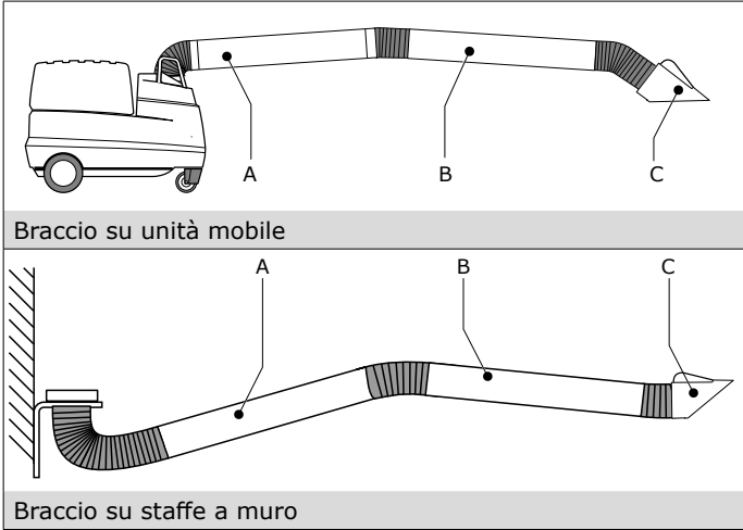
Fig. 6.1 Braccio in posizione orizzontale
