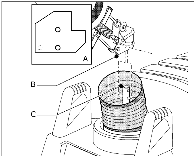
Abb. 4.3 Absaugarm auf Scharnierstange
