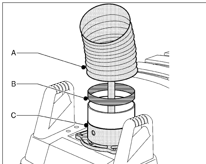
Fig. 4.2 Manguera flexible
