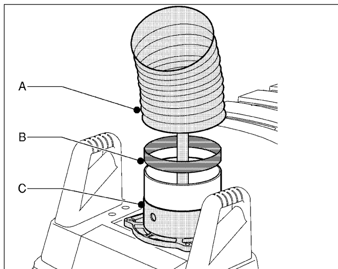
Abb. 4.2 Flexschlauch
