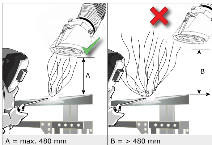
Fig. 5.2 Juiste positie van de kap
