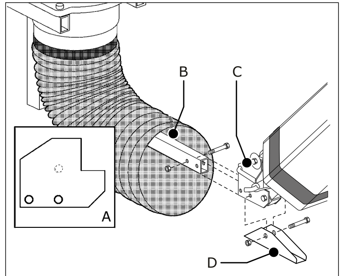
Fig. 4.6 Brazo en el adaptador colgante
