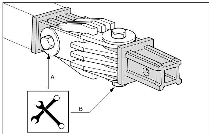
Fig. 6.2 Kapscharnier
