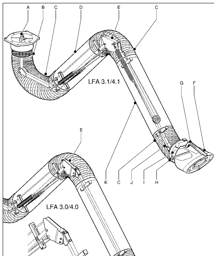
Abb. 2.1 Hauptkomponenten
