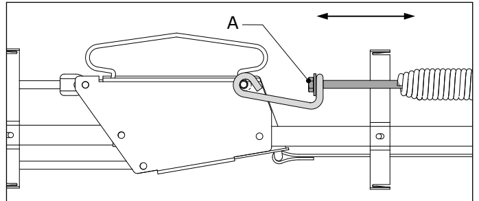
Fig. 6.4 Middle hinge – LFA 3.1 | LFA 4.1
