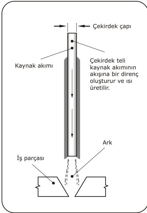
Şekil-2 Örtülü Elektrodda Kaynak Akımının İletimi
