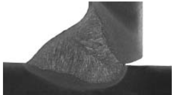
8 mm Horizontal Fillet
