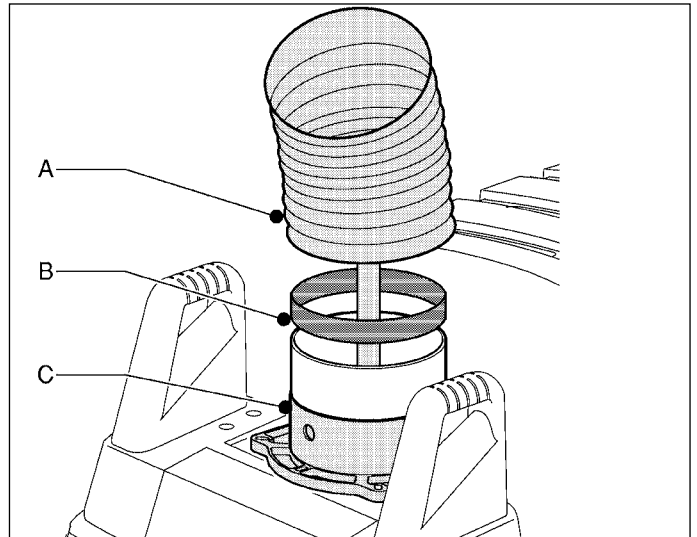
Abb. 4.2 Flexschlauch
