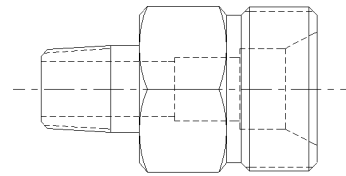
Adaptateur 9005708 pour des tuyaux collecteurs de chaque côté
